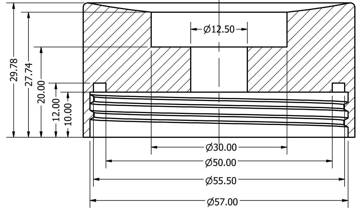
剖视图 B-B 比例 2:1
