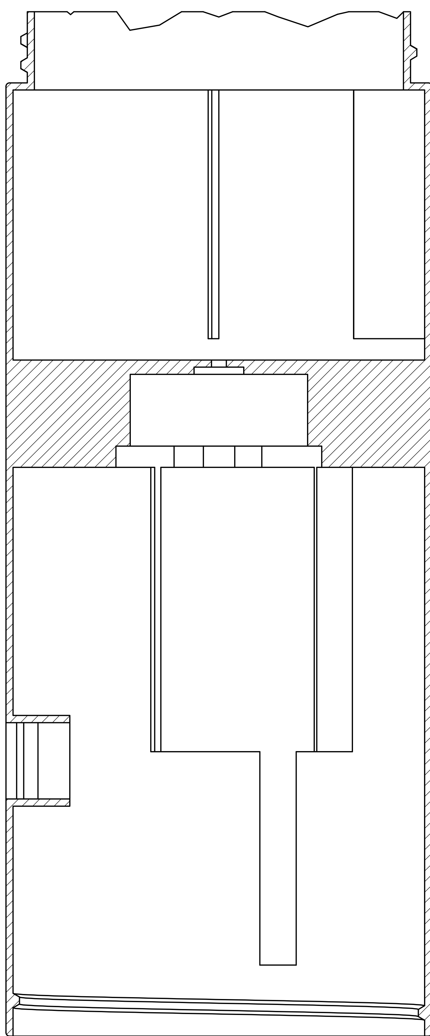
剖视图 A-A 比例 3:1
